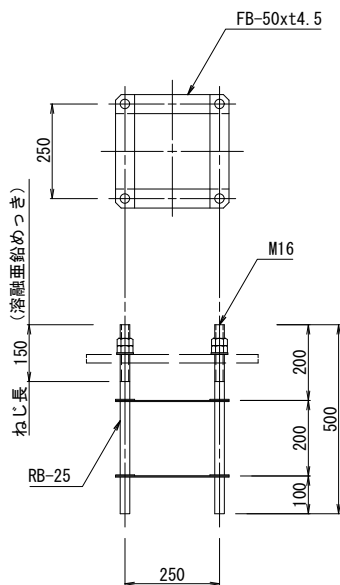
アンカーボルト詳細図 S=1:10
