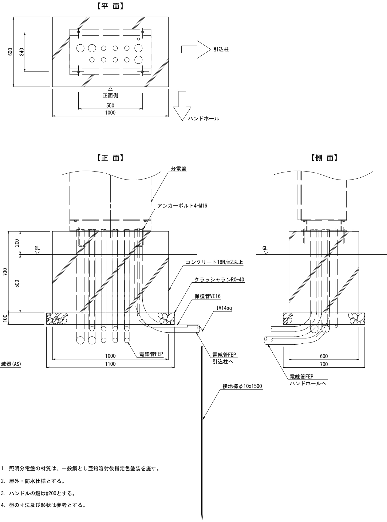
分電盤基礎詳細図
