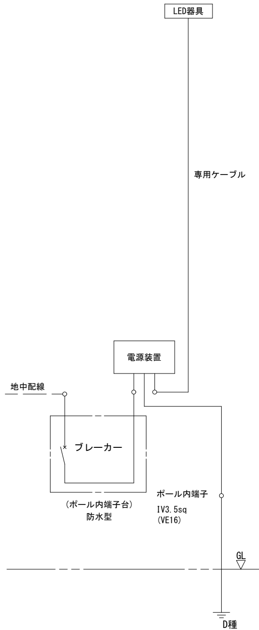
ポール内単線結線図 No scale
