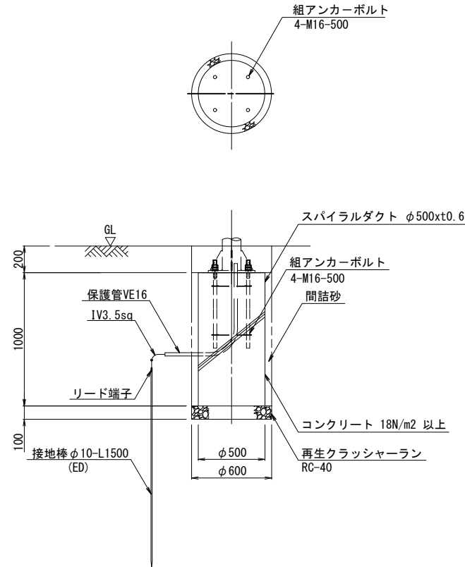
基礎詳細図 S=1:20
