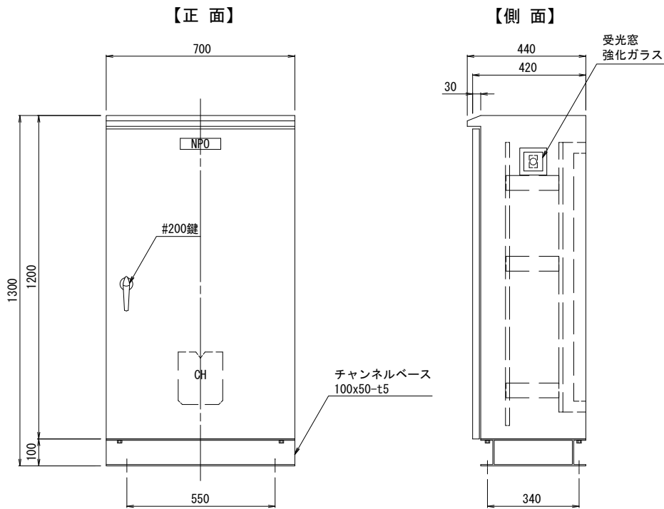
分電盤詳細図
