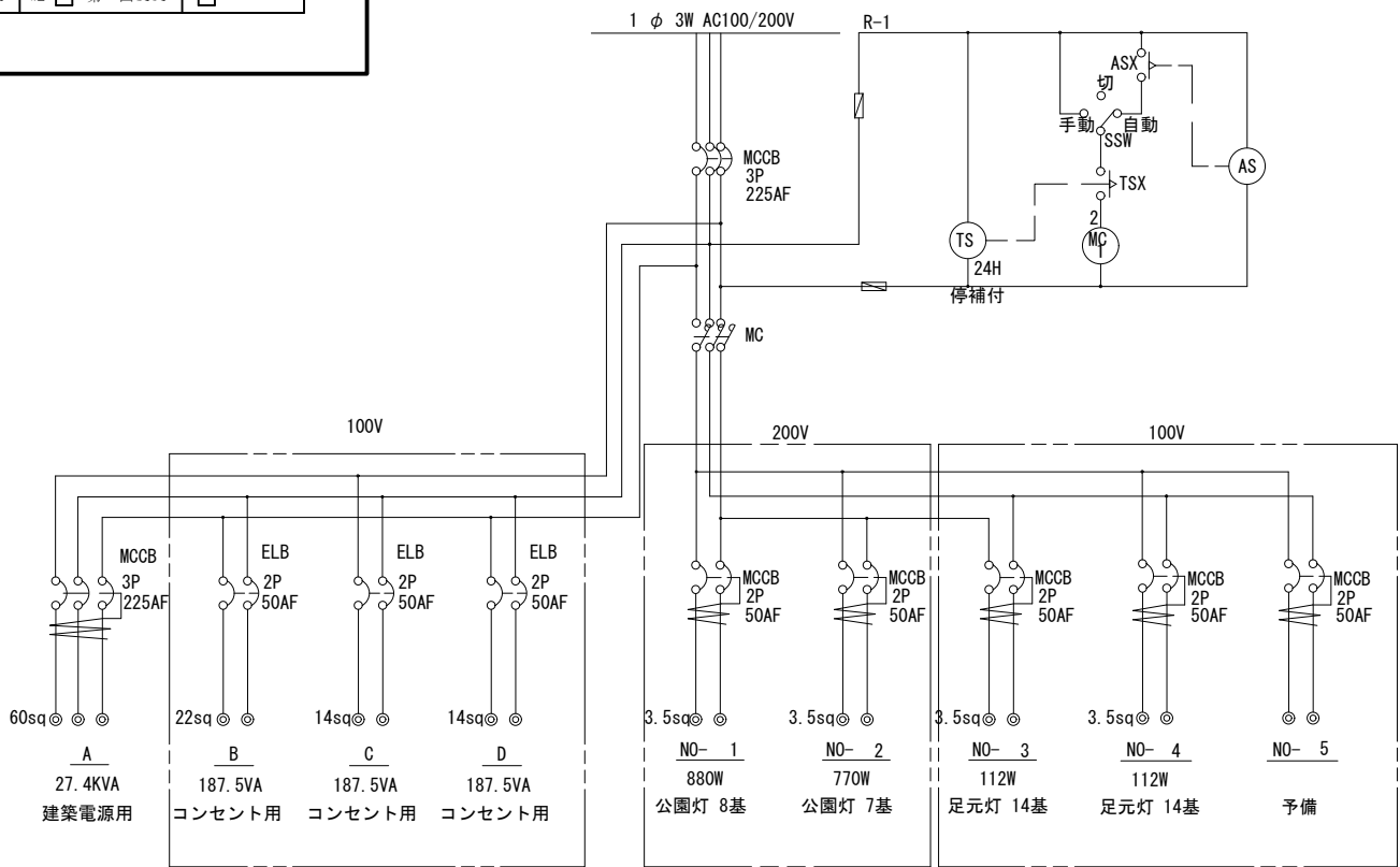
分電盤結線図
