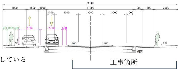
標準断面図
