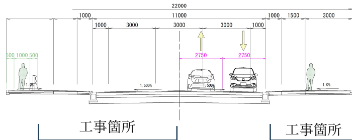
標準断面図
