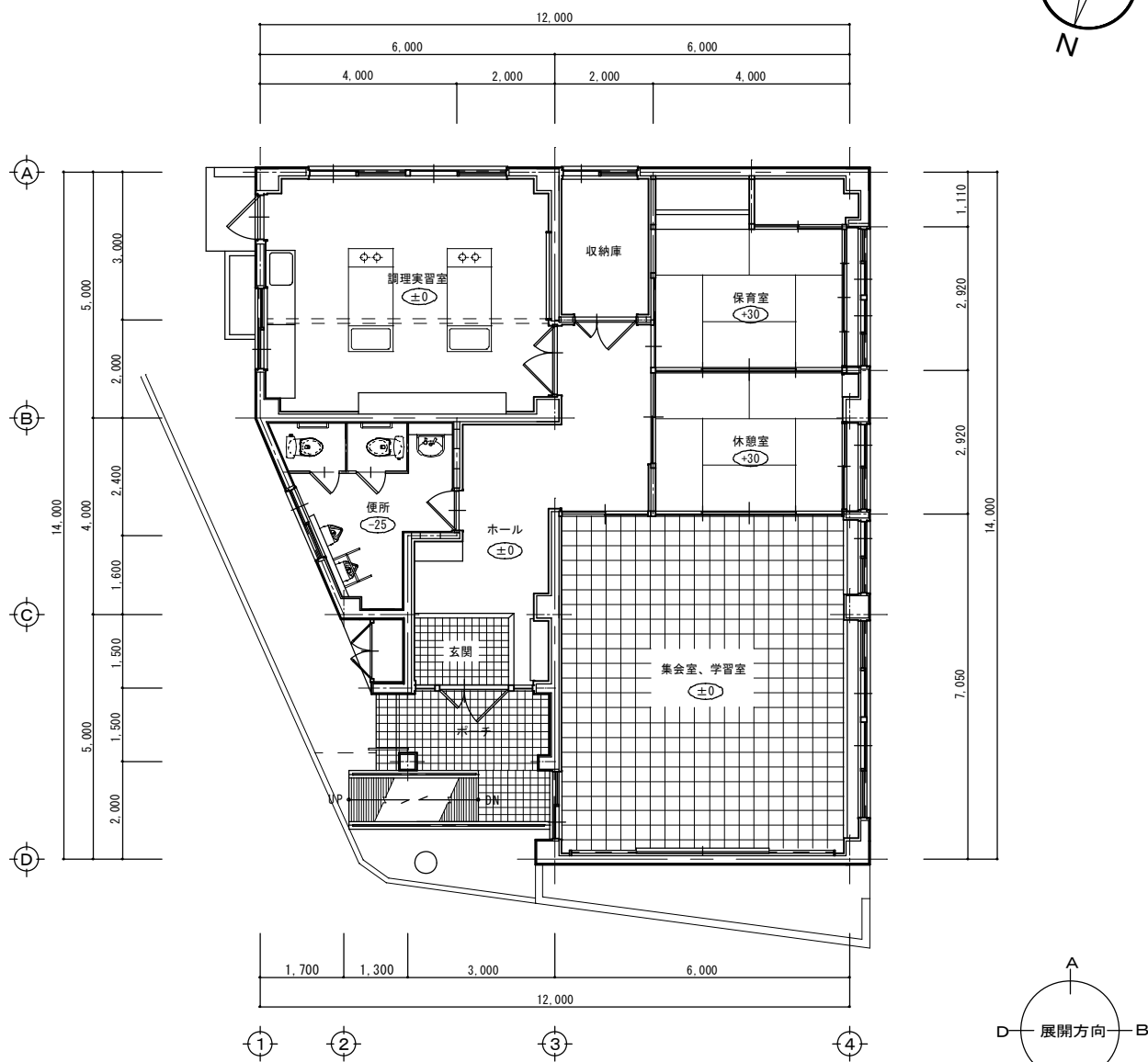
改修後 平面図 S = 1/100
