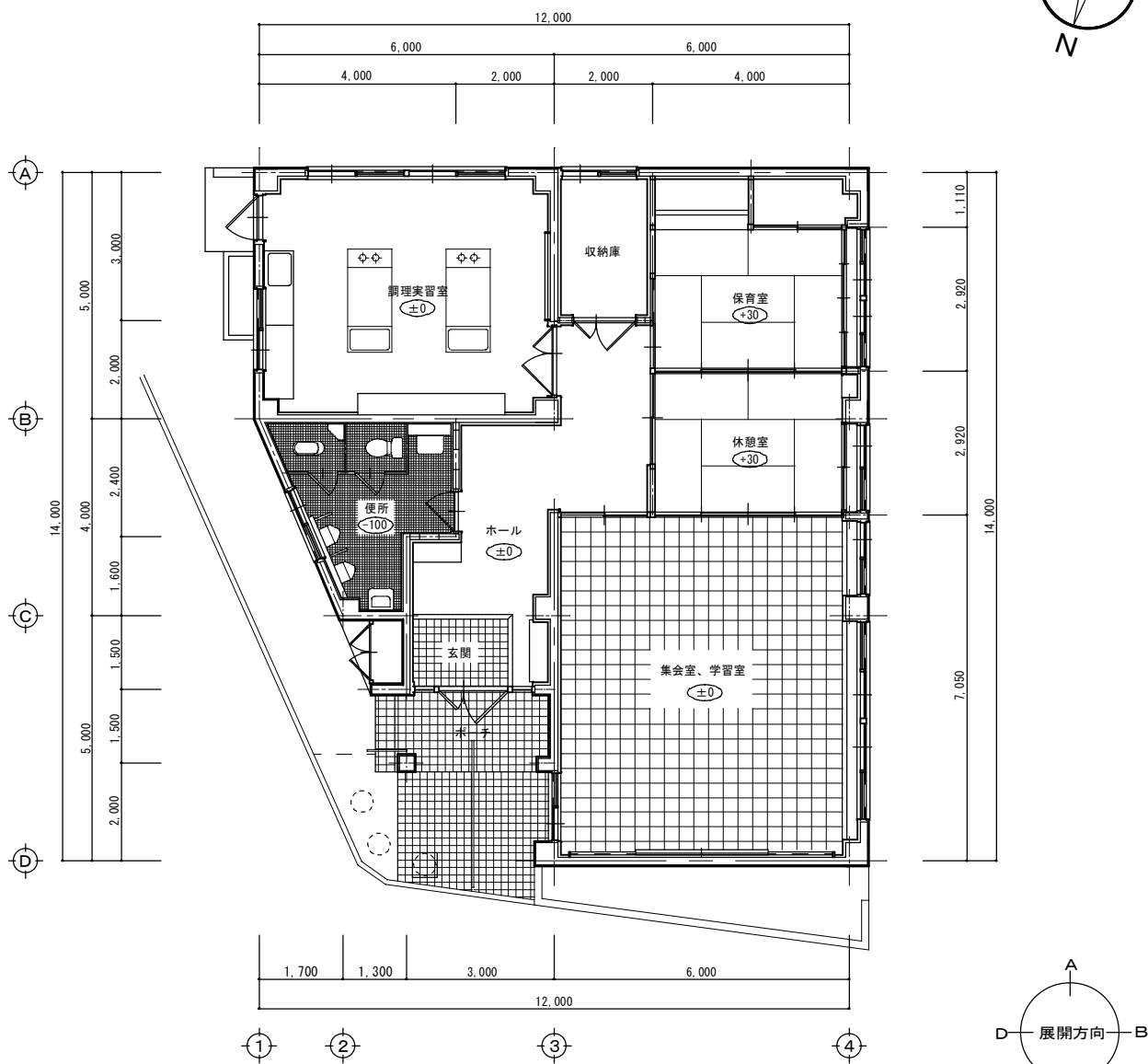
改修前 平面図 S = 1/100
