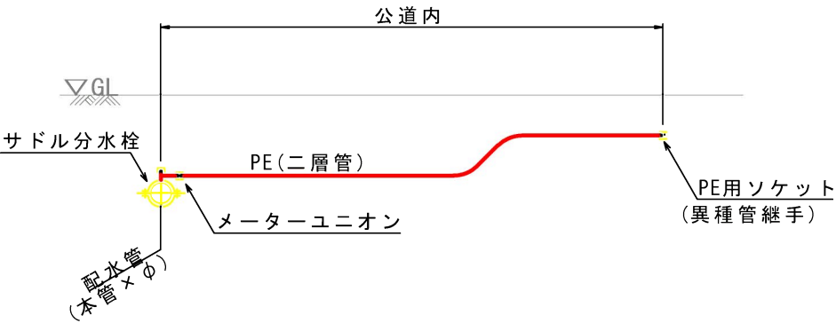
給水タイプ B
