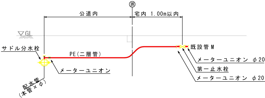
給水タイプ C
