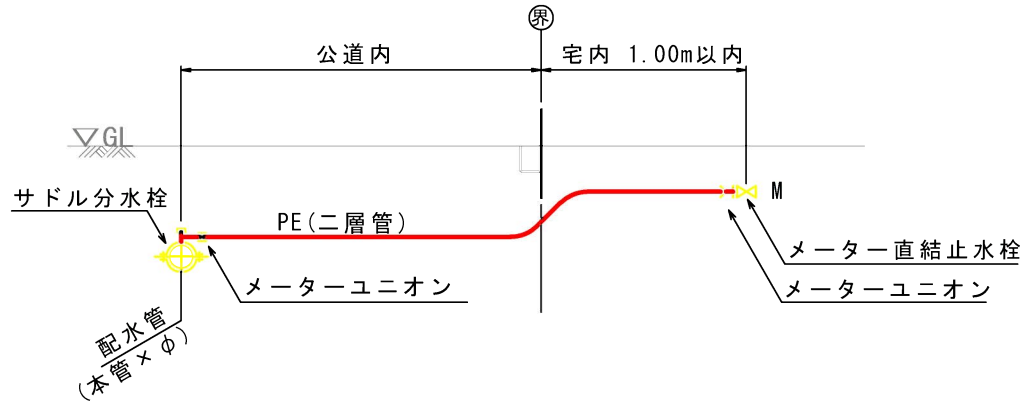
給水タイプ A
