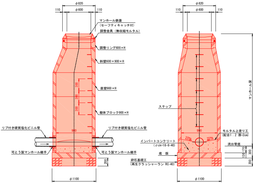
A-A断面図
