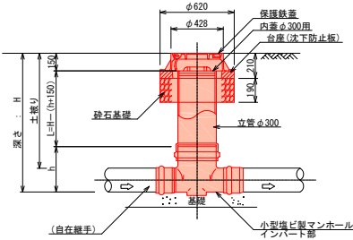
2-2断面図
