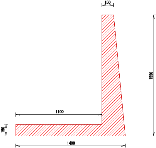
既設コンクリート撤去 S=1:100
