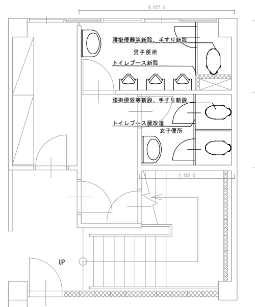
西棟 2階平面図
