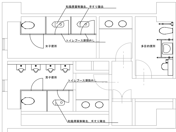
東棟 7階平面図
