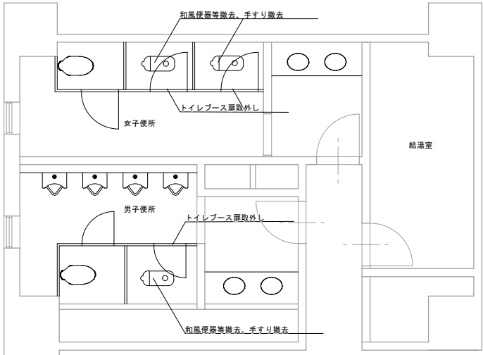
東棟 2・3階平面図
