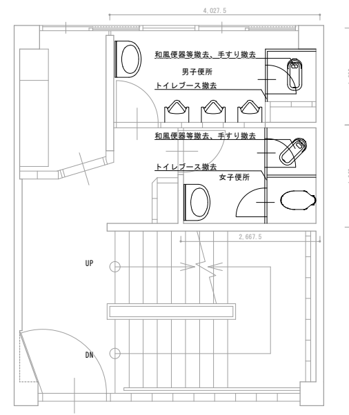
西棟 3階平面図
