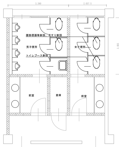
西棟 1 階平面図
