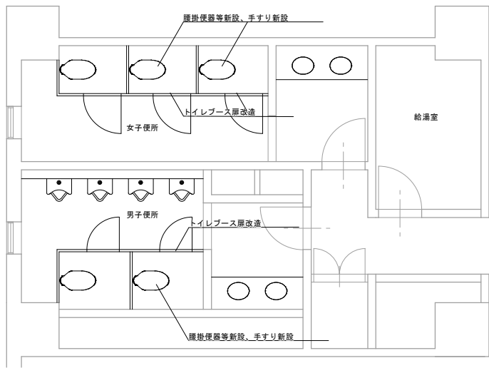
東棟 4～6階平面図
