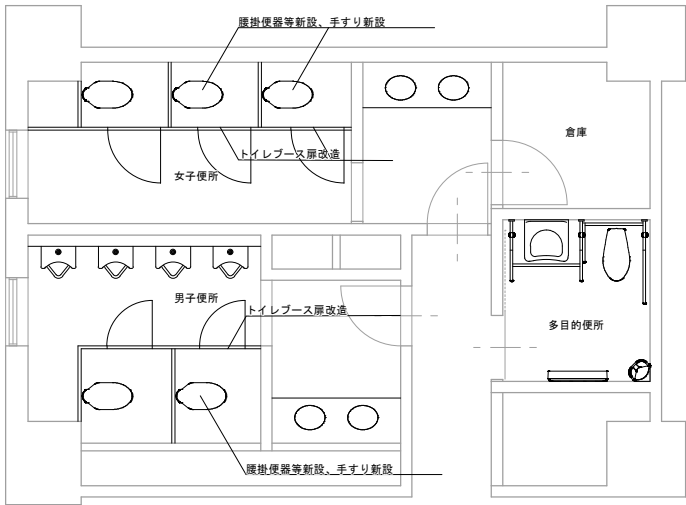
東棟 1階平面図
