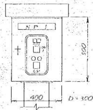
屋外自立形
