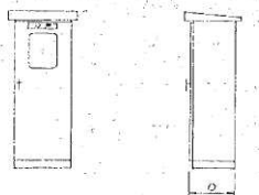
屋外自立形 正面図 側面図
